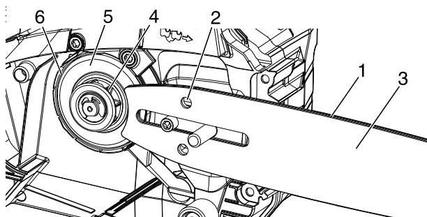
1. Rainure 2. Trou de graissage 3. Guide-chaîne
