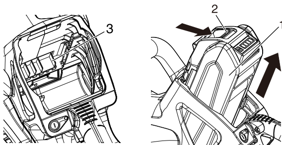
1. Batería 2. Pestillo de la batería
