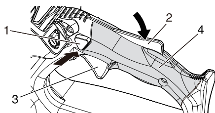
1. Fermo interruttore a grilletto 3. Interruttore a grilletto 2. Leva di rilascio fermo 4. Superficie di presa
