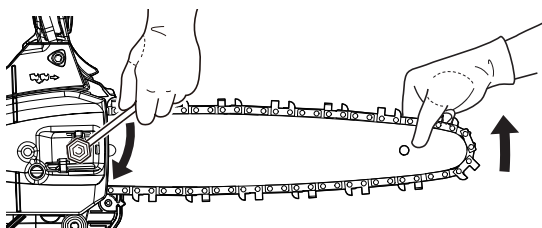
1. Tendeur de chaîne 2. Sens de tension de la chaîne
