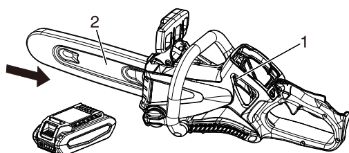
1. Scomparto batterie
