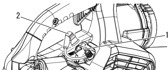
1. Zündkerze
