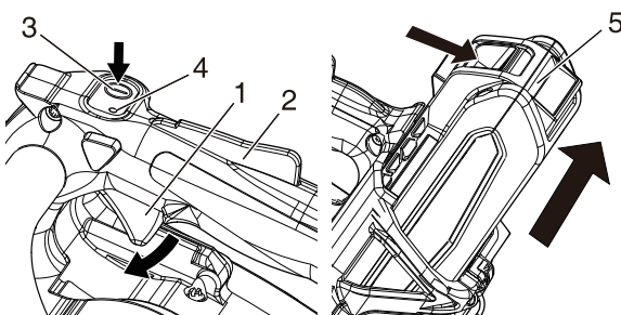
1. Hebelschalter 2. Sperrenlösehebel 3. Ein/Aus-Knopf
