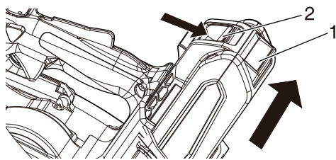
2. Fermo del pacco batterie
