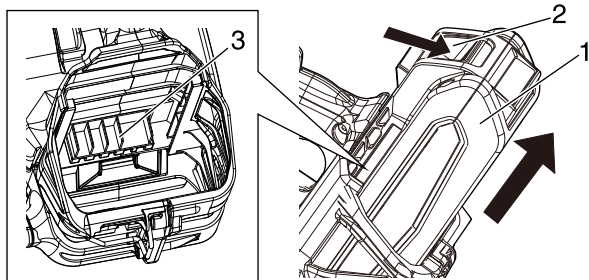
1. Batterie 2. Verrou de la batterie
