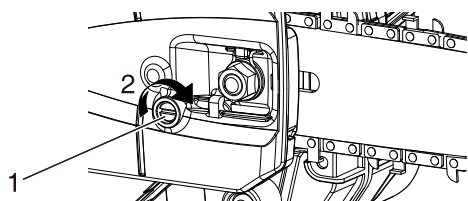
1. Tendicatena 2. Direzione per tendere la catena
