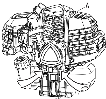
Luftzufuhröffnung
