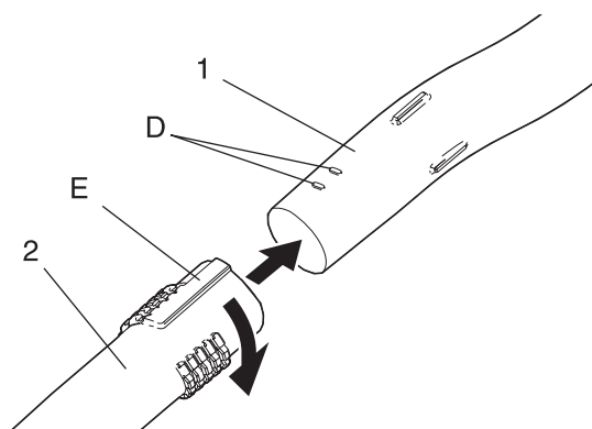
1. Tubo del soffiatore
