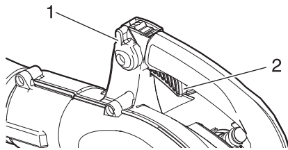
1. Leva di regolazione del gas 2. Leva dell'acceleratore
