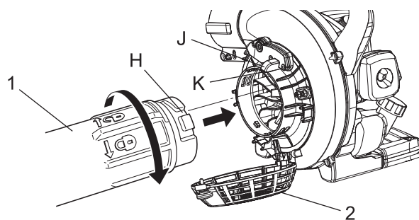
1. Tubo de vacío
