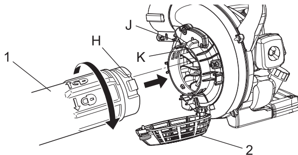
1. Tube d'aspiration
