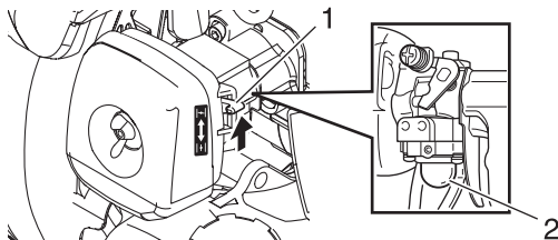
1. Valvola dell'aria 2. Bulbo di spurgo
