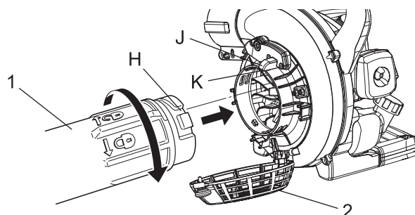
1. Saugrohr
