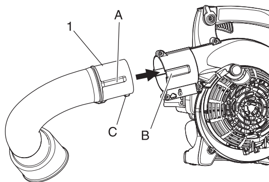
1. Saugrohr-Bogenstück
