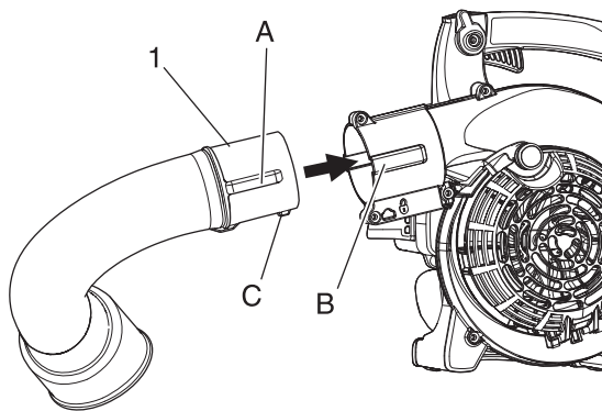
1. Coude d'aspiration
