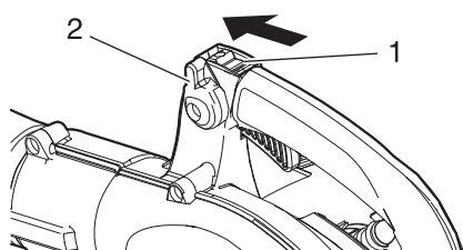
1. Interruptor de paro 2. Palanca de posición del acelerador
