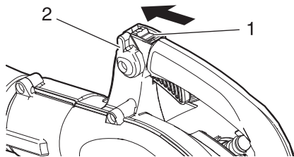
1. Interruttore di arresto 2. Leva di regolazione acceleratore
