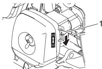
1. Estárter por retroceso
