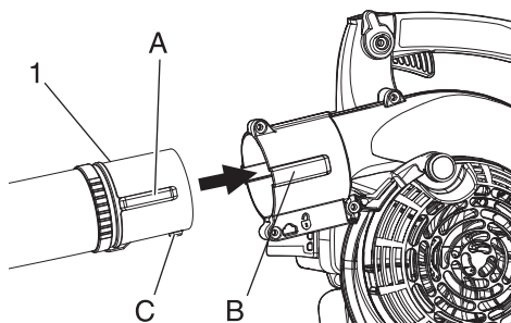
1. Tubo del soplador
