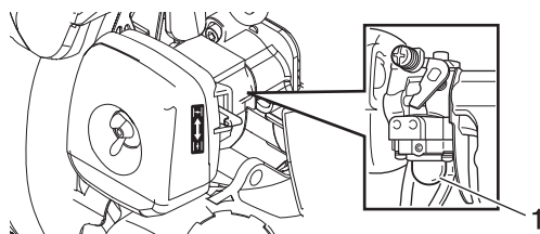
1. Kraftstoffpumpe
