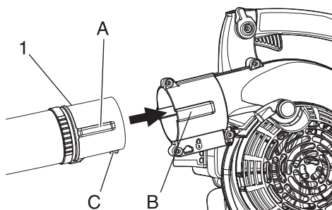
1. Tubo del soffiatore
